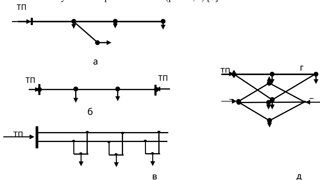
Рисунок 2. Характерные однолинейные схемы электрических сетей
