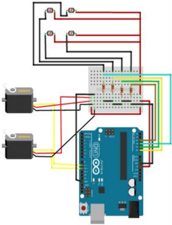
Рис.5. Схема соединения технологического процесса с Arduino.
