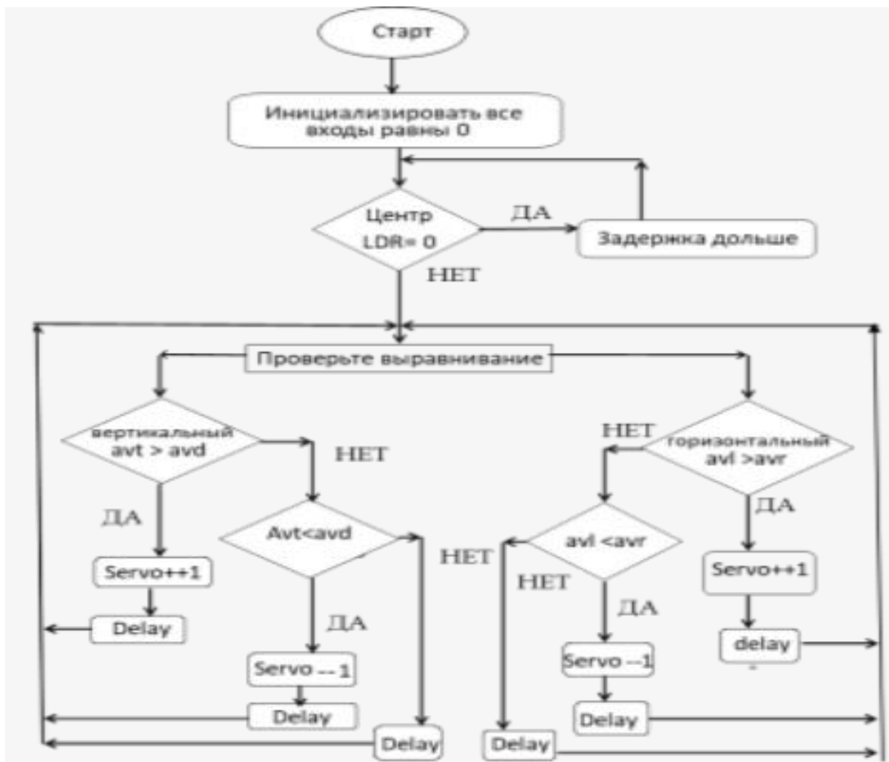
Рис.6. Алгоритм управления солнечного коллектора.
