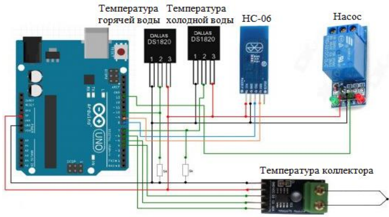
Рис.7. Схема регулирования температуры солнечного коллектора.
