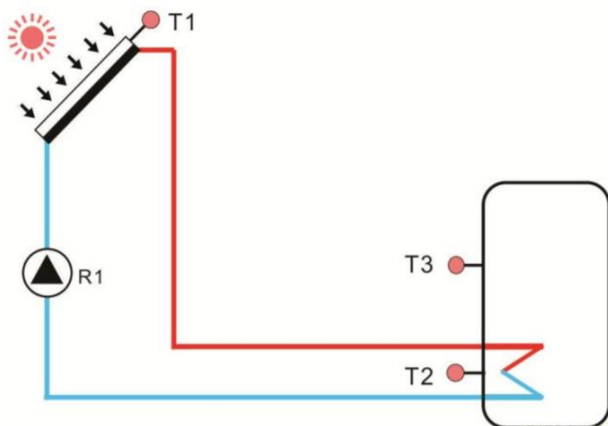
Рис.4. Структурная схема солнечного коллектора.
