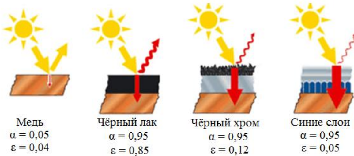
Рис.2. Зависимость теплового отражения от поверхности материала.
