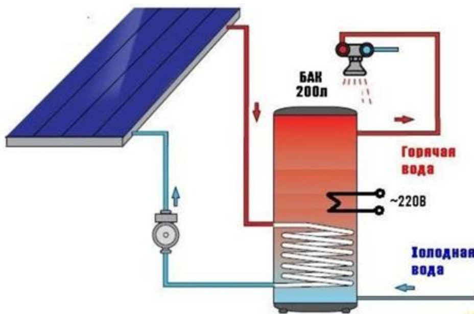
Рис.3. Функционально-технологическая схема солнечного коллектора.
