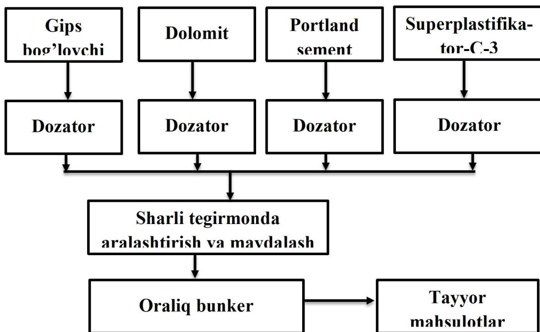
1-rasm - Gips va sement ishlab chiqarishning texnologik sxemasi putssolan birikmasi.
